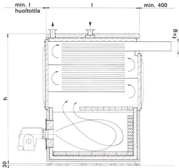
Öljy- tai kaasukäyttöinen ylipaineekattila.
