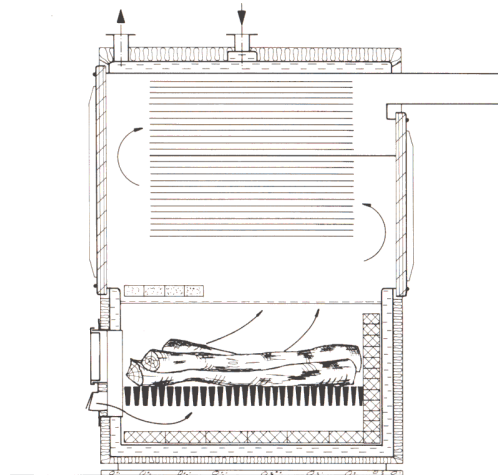
Luonnonvetoinen alipaineekattila.
